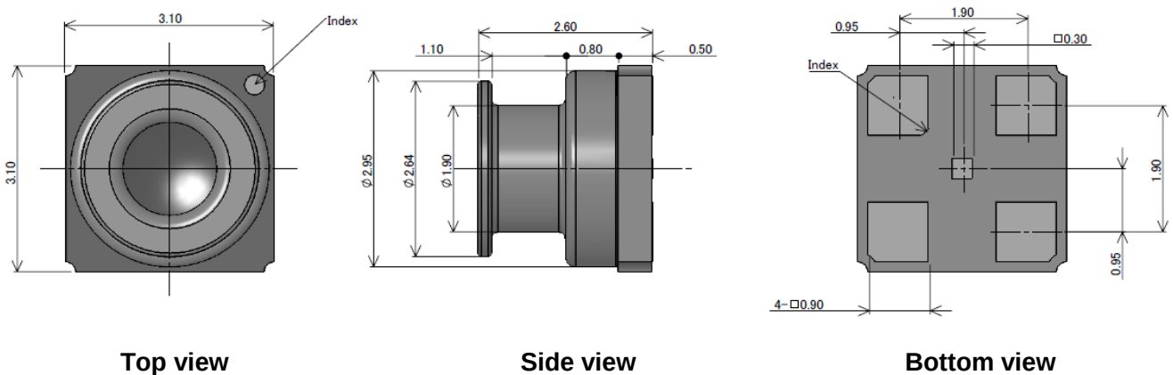
Fig. 16 : Mechanical Dimension
