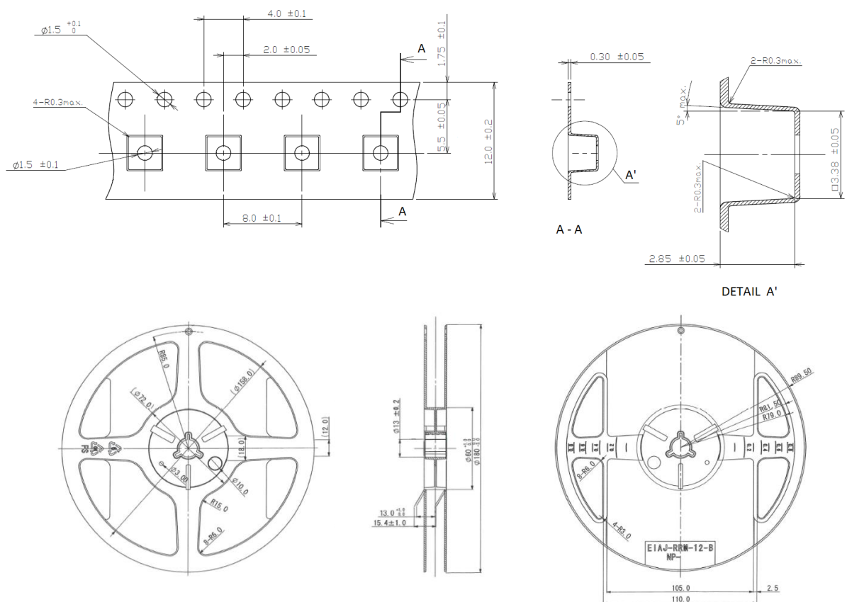
Fig. 18 : Tape and Reel dimension
